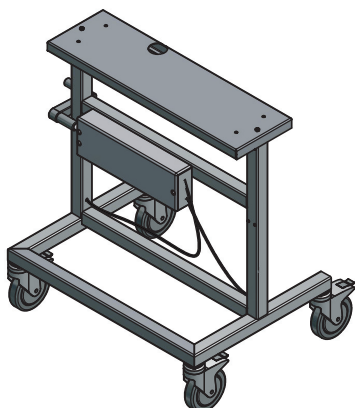
Hev senk understell til sveiselist
